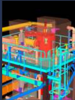
COALESCER MODULE SKID
